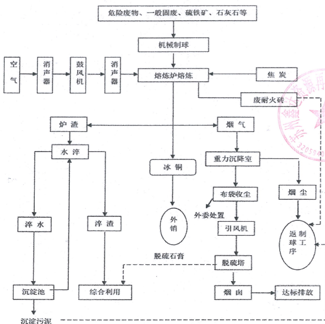
1-1 项目工艺流程示意图
